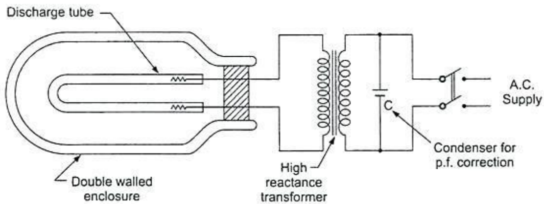
Fig. 7 Sodium vapour lamp
